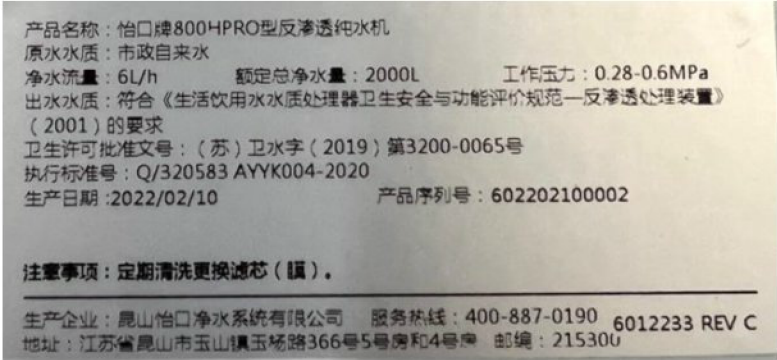
800HPRO（铭牌）
